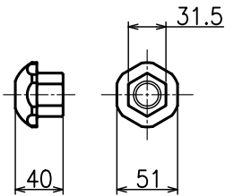
③ 球面ナット
