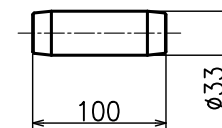
⑧ カプラー
