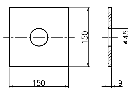
⑦ スペーサー
