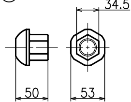
③ 球面ナット
