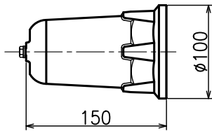
② アルミキャップ (アルミ合金) ※グリス入り
