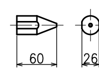
⑨ 先端キャップ ※現場組込み
