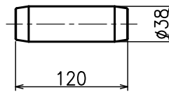
⑧ カプラー
