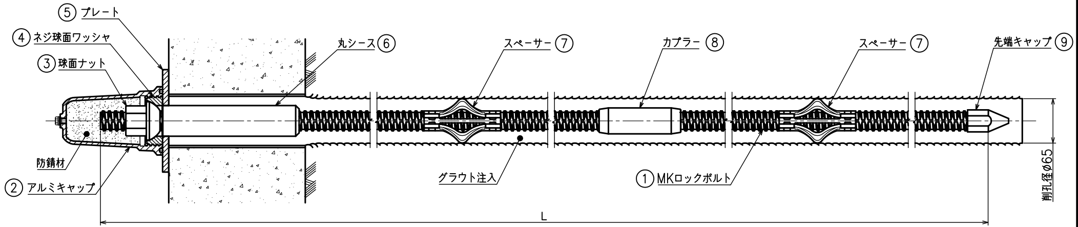
⑤ プレート
