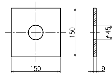
⑨ 先端キャップ ※現場組込み
