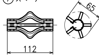
⑦ スペーサー
